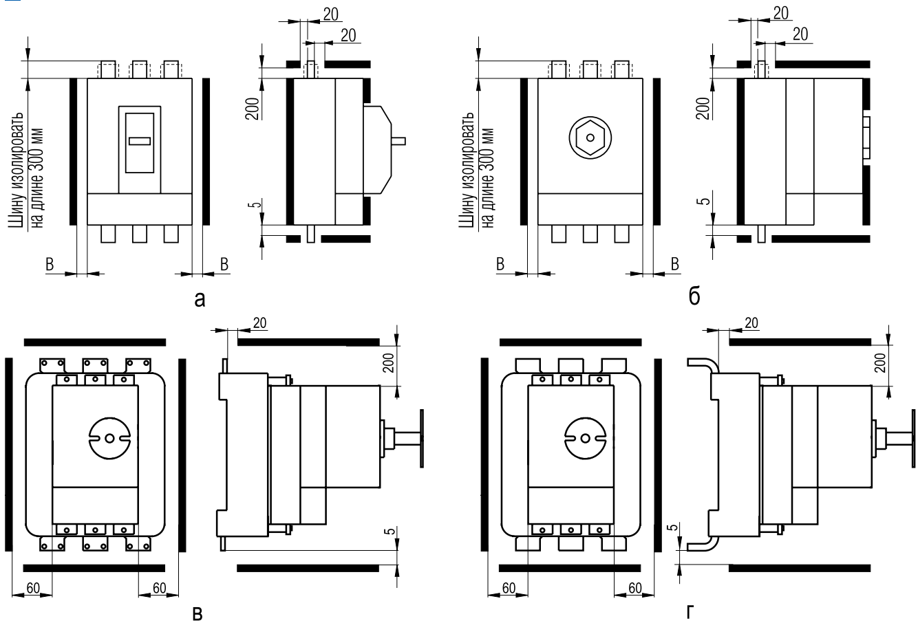
Рисунок В.12. Минимальные расстояния от металлических частей распреустройства до выключателей
