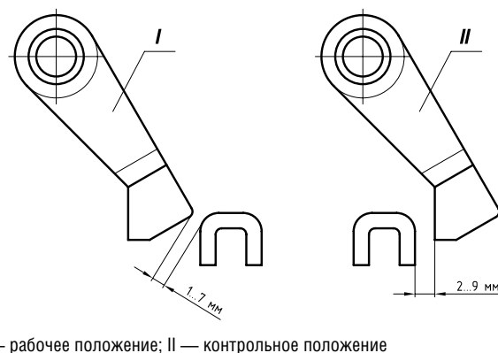
Рисунок 15. Механическая блокировка выключателей Э16В, Э25В, Э40В
