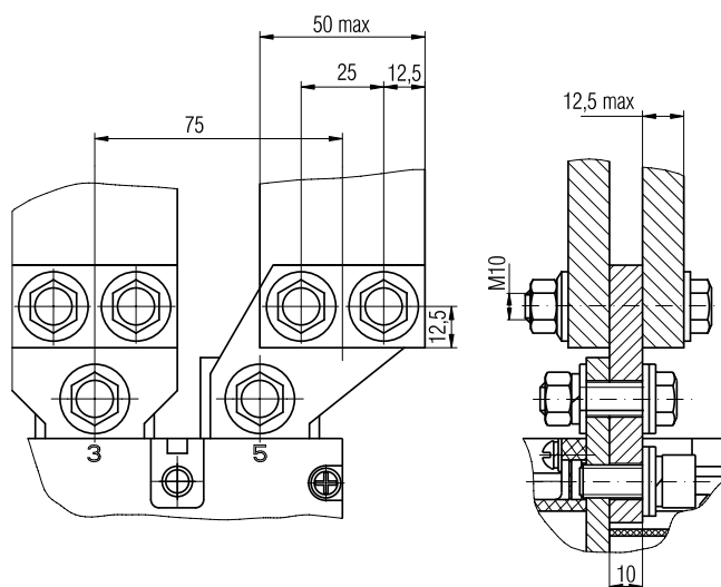
Рисунок Б.6. Переднее присоединение шиной или двумя шинами «плашмя» с переходником или кабелями (1-4) с кабельным наконечником ГОСТ 7387-82, ГОСТ 7386-80, с контактным стержнем \varnothing 10 мм для выключателей типа ВА08-040Х, ВА08-063Х, ВА08-080Х (остальное см. рисунки А.1, А.2)
