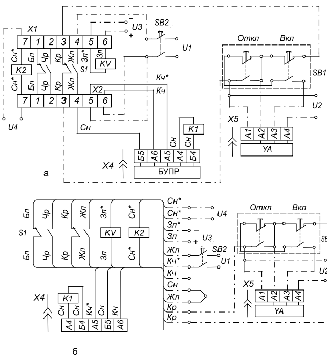
Рисунок 34. Схема электрическая соединений дополнительных сборочных единиц выключателей стационарного исполнения АЗ793Б, АЗ794Б
