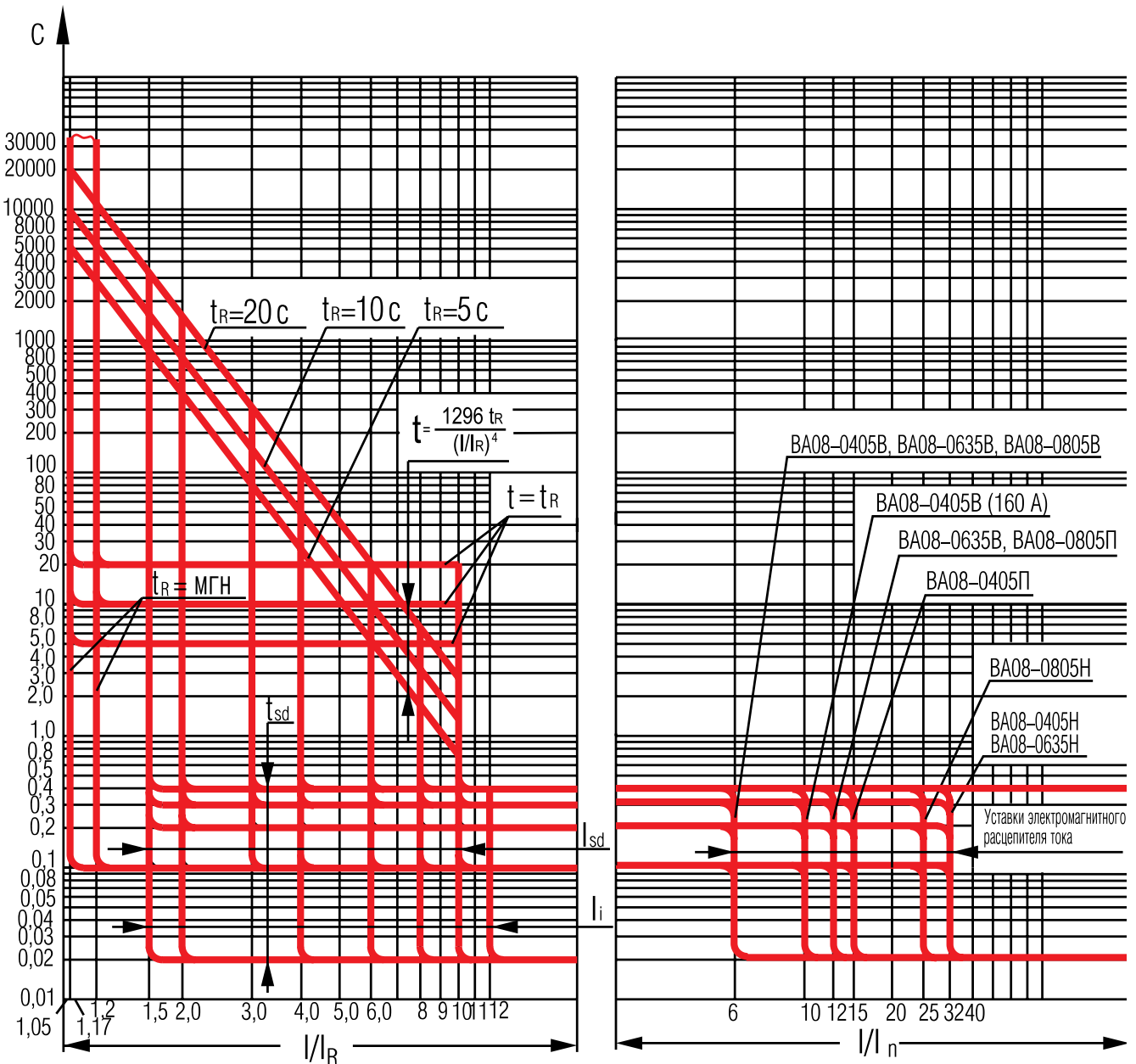
Рисунок Г.8. Временная характеристика выключателя переменного тока с полупроводниковым (микропроцессорным) расцепителем тока и электромагнитным расцепителем тока
