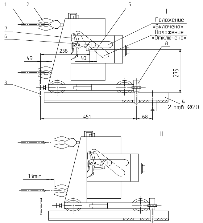
Рисунок 12а. Выключатели выдвигного исполнения АВ2М15, АВ2М20
