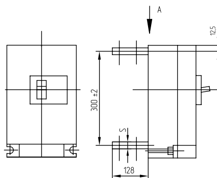
Рисунок А.3. Выключатели типов ВА52-41, ВА53-41, ВА55-41, ВА56-41 стационарного исполнения с ручным приводом для заднего присоединения
