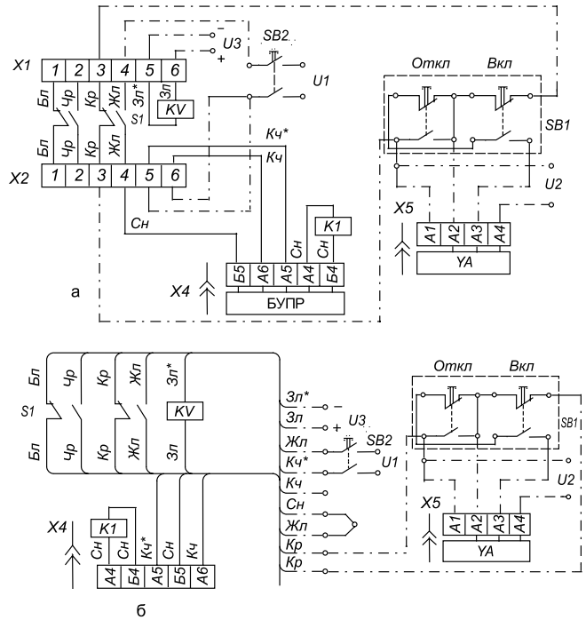
Рисунок 35. Схема электрическая соединений дополнительных сборочных единиц выключателей стационарного исполнения АЗ794Б, АЗ793С, АЗ794С
