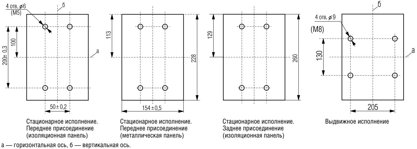
Рисунок 12. Отверстия в панели для установки выключателей
