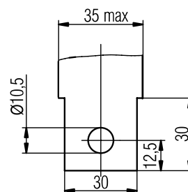
Рисунок Б.6. Переднее присоединение шиной или двумя шинами «плашмя» с переходником или кабелями (1-4) с кабельным наконечником ГОСТ 7387-82, ГОСТ 7386-80, с контактным стержнем \varnothing 10 мм для выключателей типа ВА08-040Х, ВА08-063Х, ВА08-080Х (остальное см. рисунки А.1, А.2)
