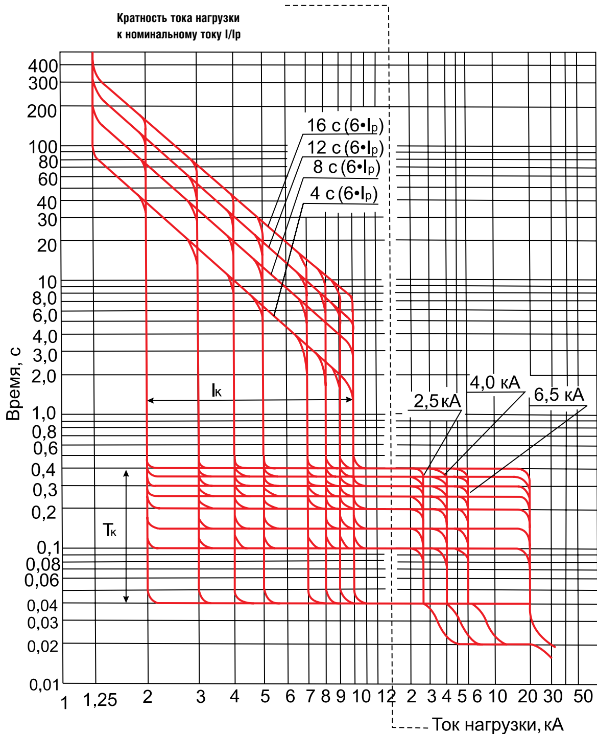
Рисунок 44. Временнoвая характеристика выключателей переменного тока А3793Б и А3793С, А3794Б и А3794С
