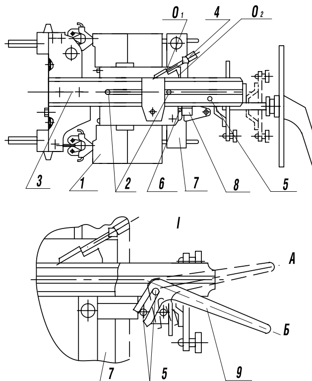
Рисунок 23. Выключатель выдвигного исполнения
