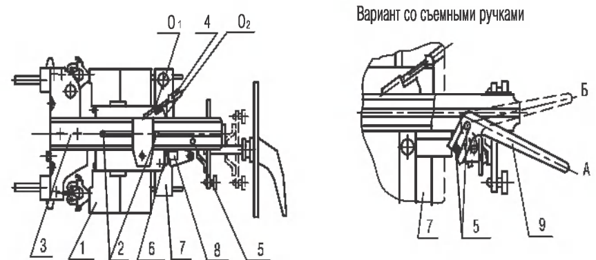
Рисунок 9 - Установка ручного привода
