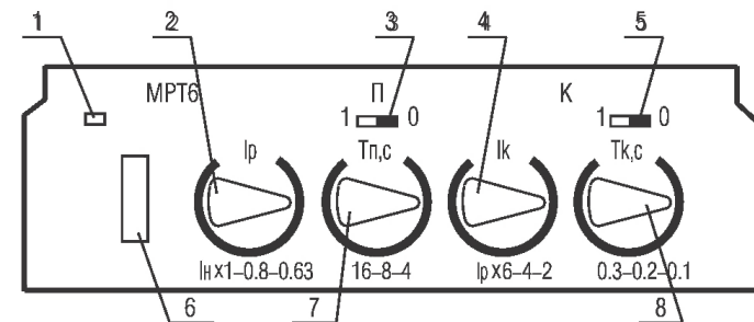
Рисунок 13 - Общий вид лицевой панели блока МРТ4-МП
