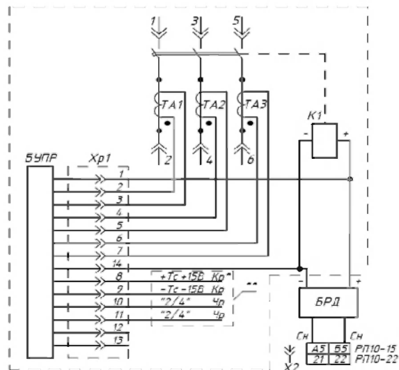
Выдвижное исполнение
