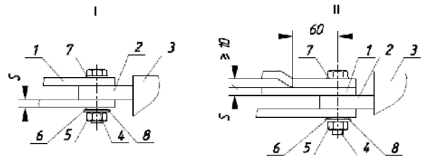
Присоединение алюминиевых шин: I – на 1600 А, II – на 2000 А
