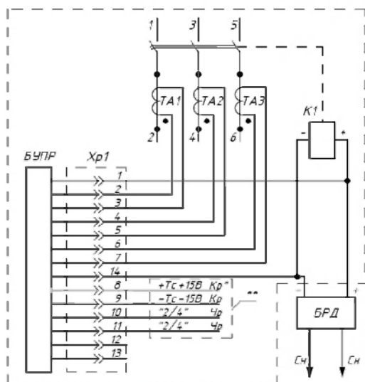
Стационарное исполнение
