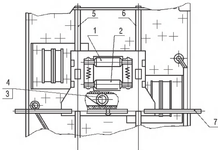
Рисунок 15 - Места смазки механизма выключателей
