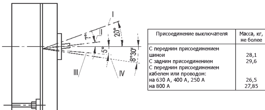
Рисунок А.1 - Выключатели типов ВА52-41, ВА53-41, ВА55-41, ВА56-41 стационарного исполнения с ручным приводом
