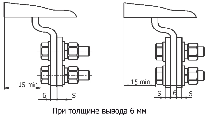
Рисунок А.8 - Способы присоединения внешних проводников к выключателям с передним присоединением
