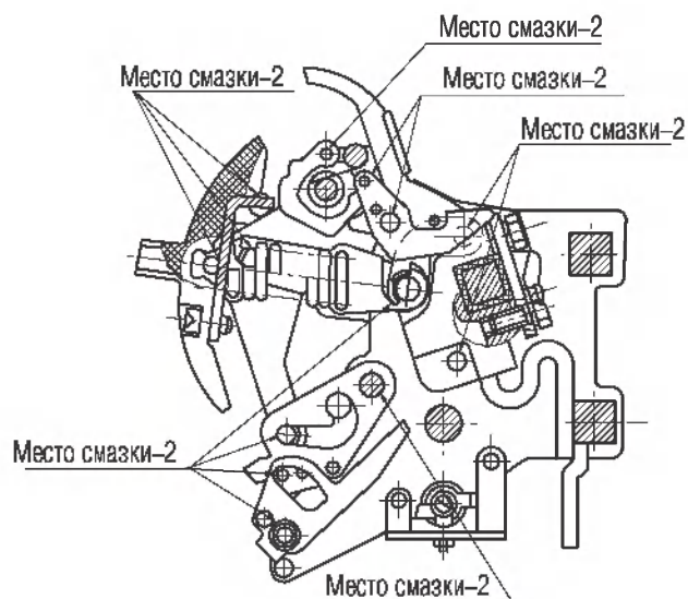
Рисунок А.20 - Места смазки механизма выключателей
