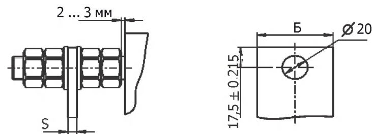
Присоединение шпилькой
